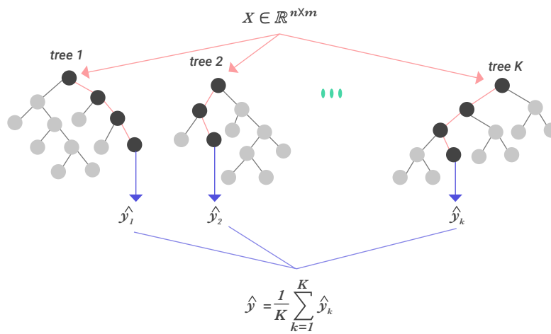
Figura 27. Funcionamiento de los modelos basados en múltiples árboles de decisión.
