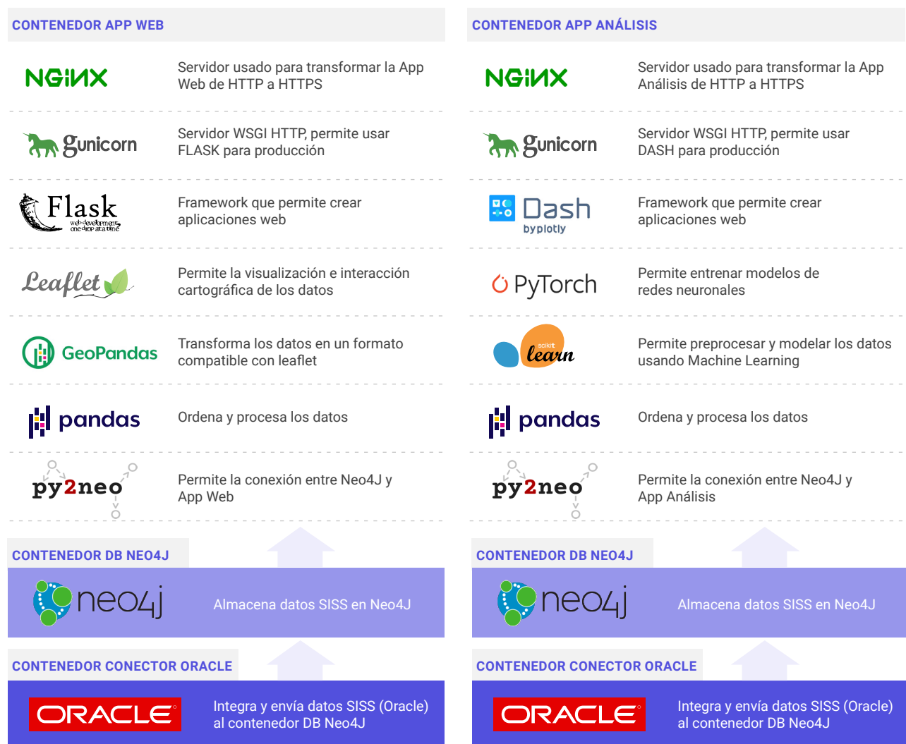
Figura 15. Mecanismo de operación e implementación del contenedor de la aplicación web y de la aplicación de análisis.
