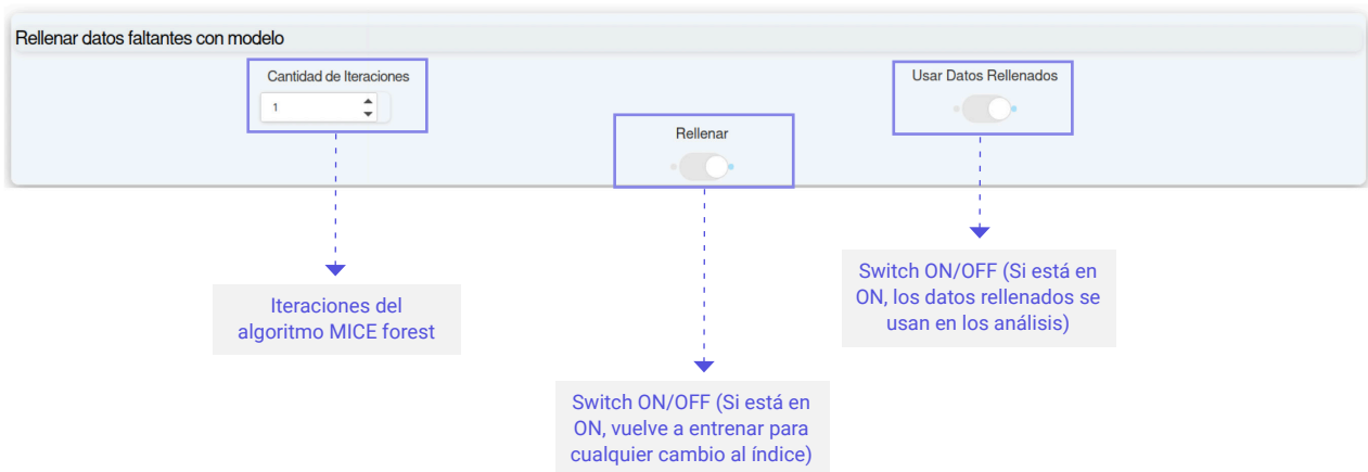
Figura 26. Uso del algoritmo de rellenado de datos en la aplicación de análisis.
