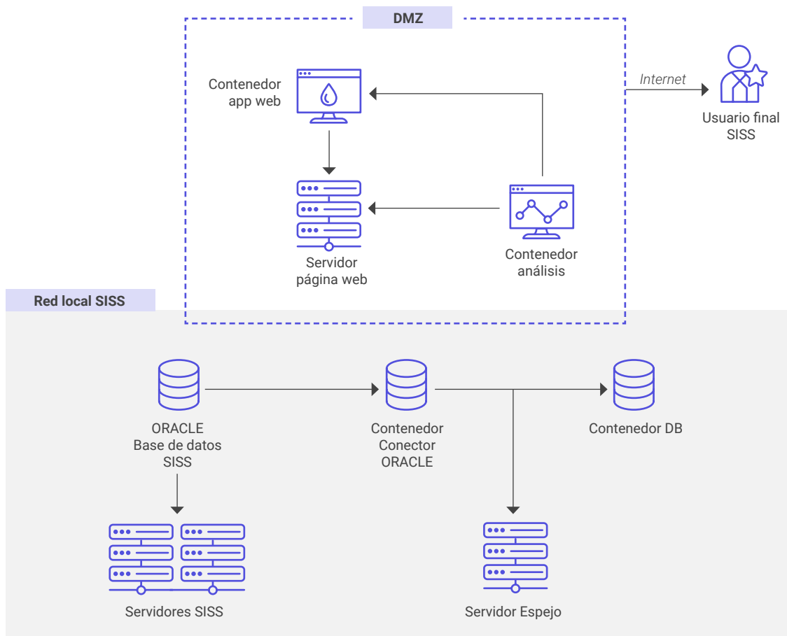
Figura 14. Diagrama de implementación del sistema en base a contenedores y dos servidores en las dependencias de la SISS.
