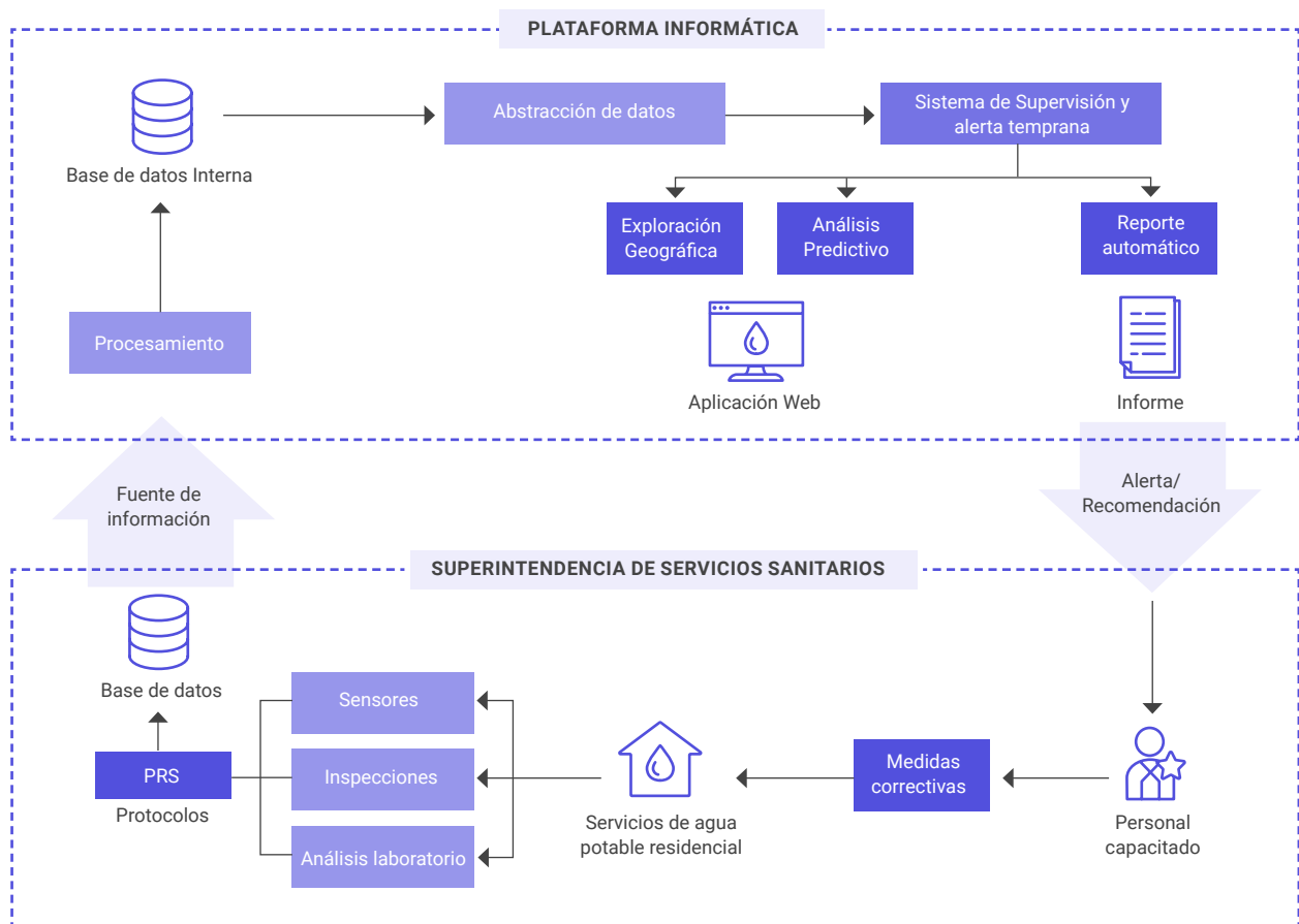
Figura 12. Concepto de operación del SSAT prototipo en el contexto actual de la SISS.
