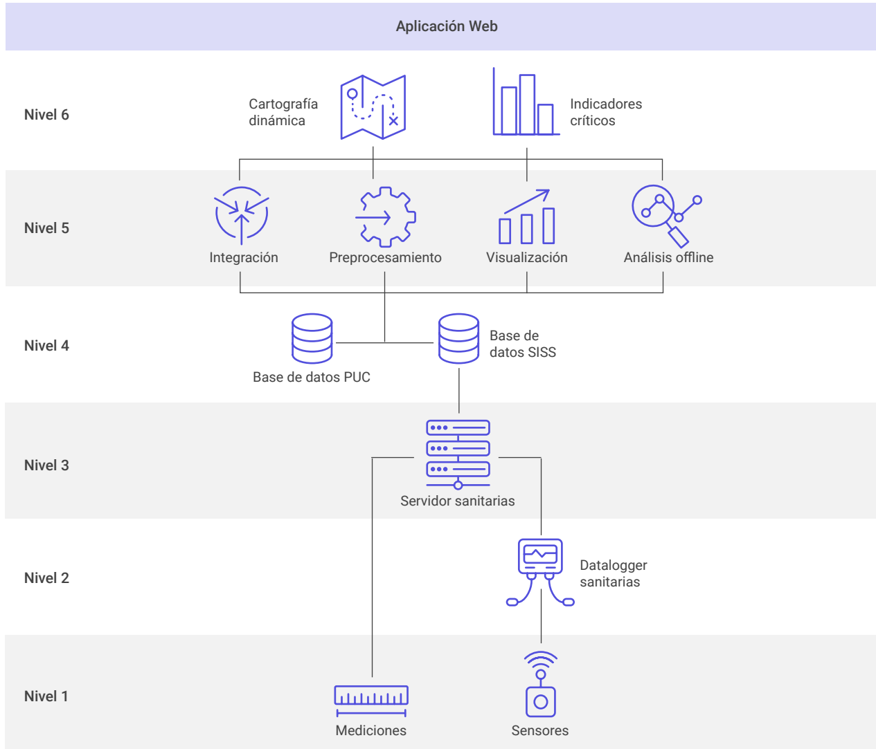
Figura 13. Diseño conceptual del sistema de monitoreo en base al modelo de referencia IoT World Forum.
